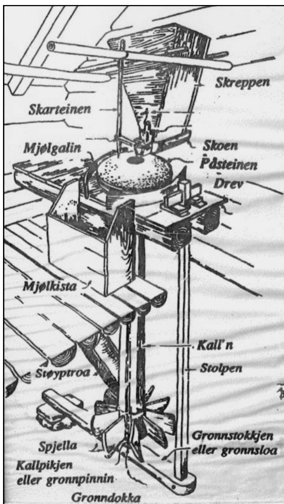
Tegning av en typisk gårdskvern med navn brukt i Trøndelag (Egge Museum). Tegnet av Arne Berg.
