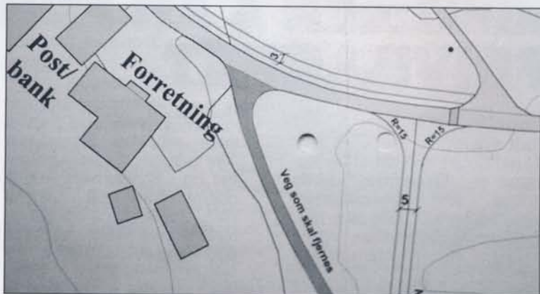
På tegningen ser du hvordan det nye vegkrysset ser ut.
