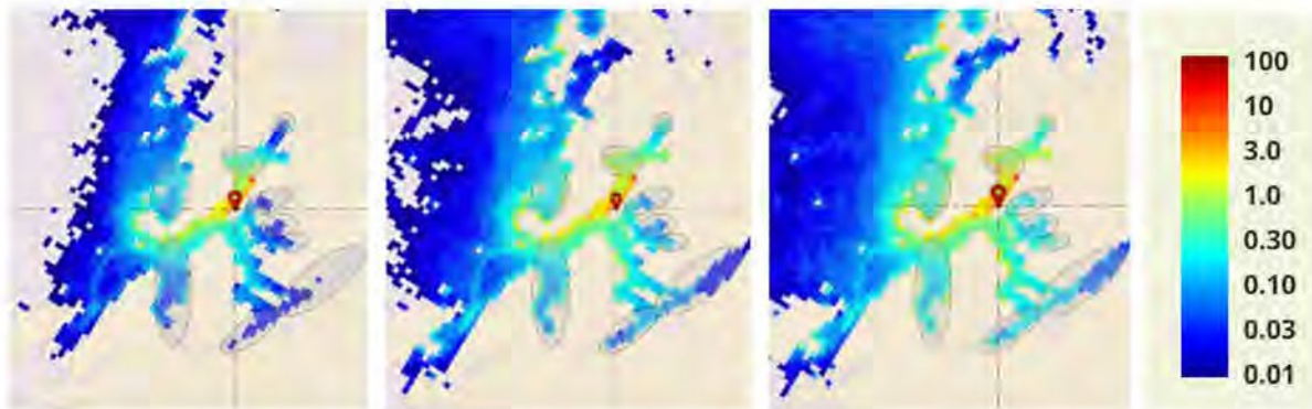
Figur 6: Strømsimulering lokalitet Farnes i ROMS-modell Nor Kyst 800 – 10, 20 og 30 dagers drift
